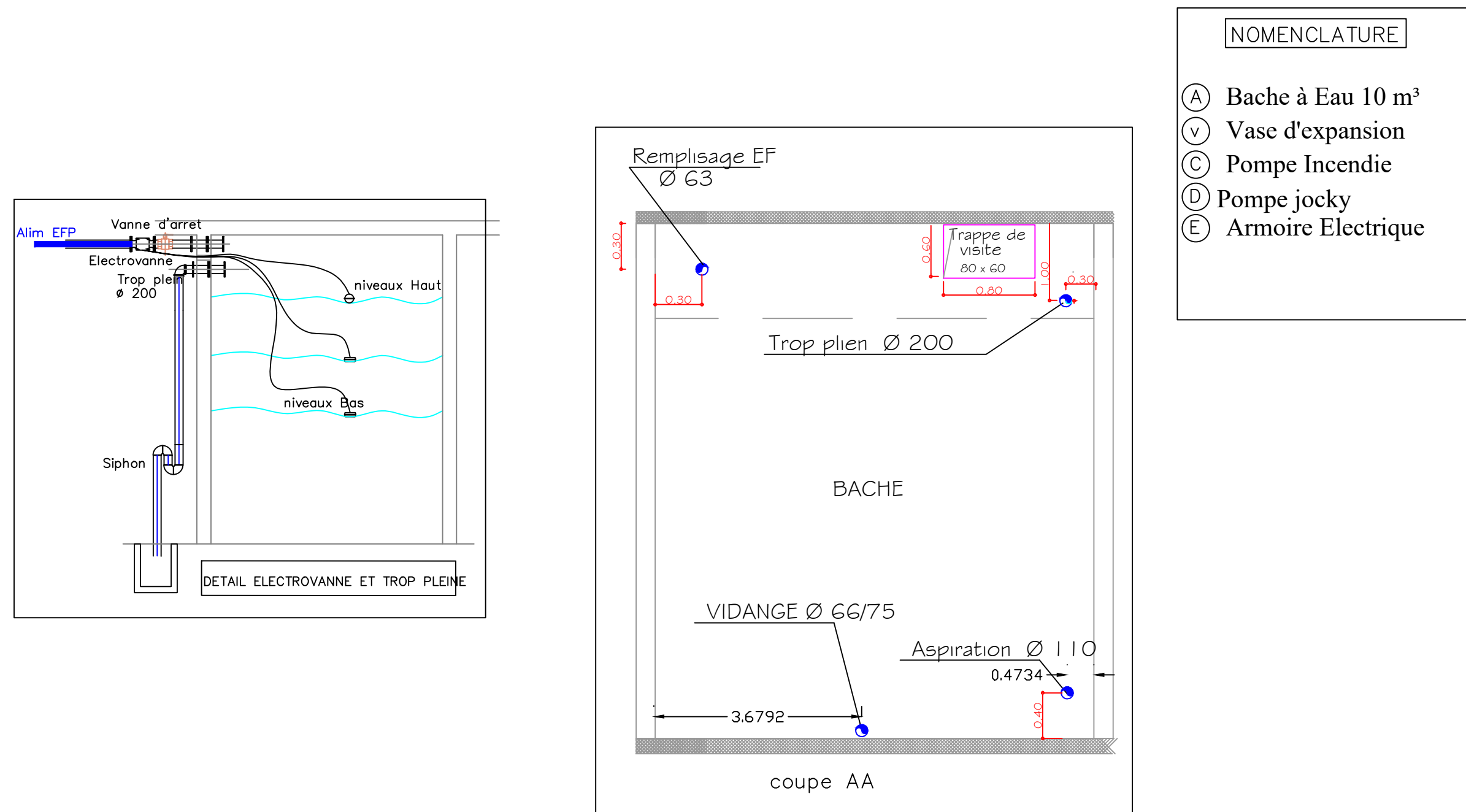
PLAN STATION DE SURPRESSION Bache à eau + Local Technique
